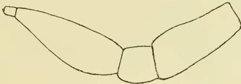
Fig. 1. Fühler ♂ 53:1.
